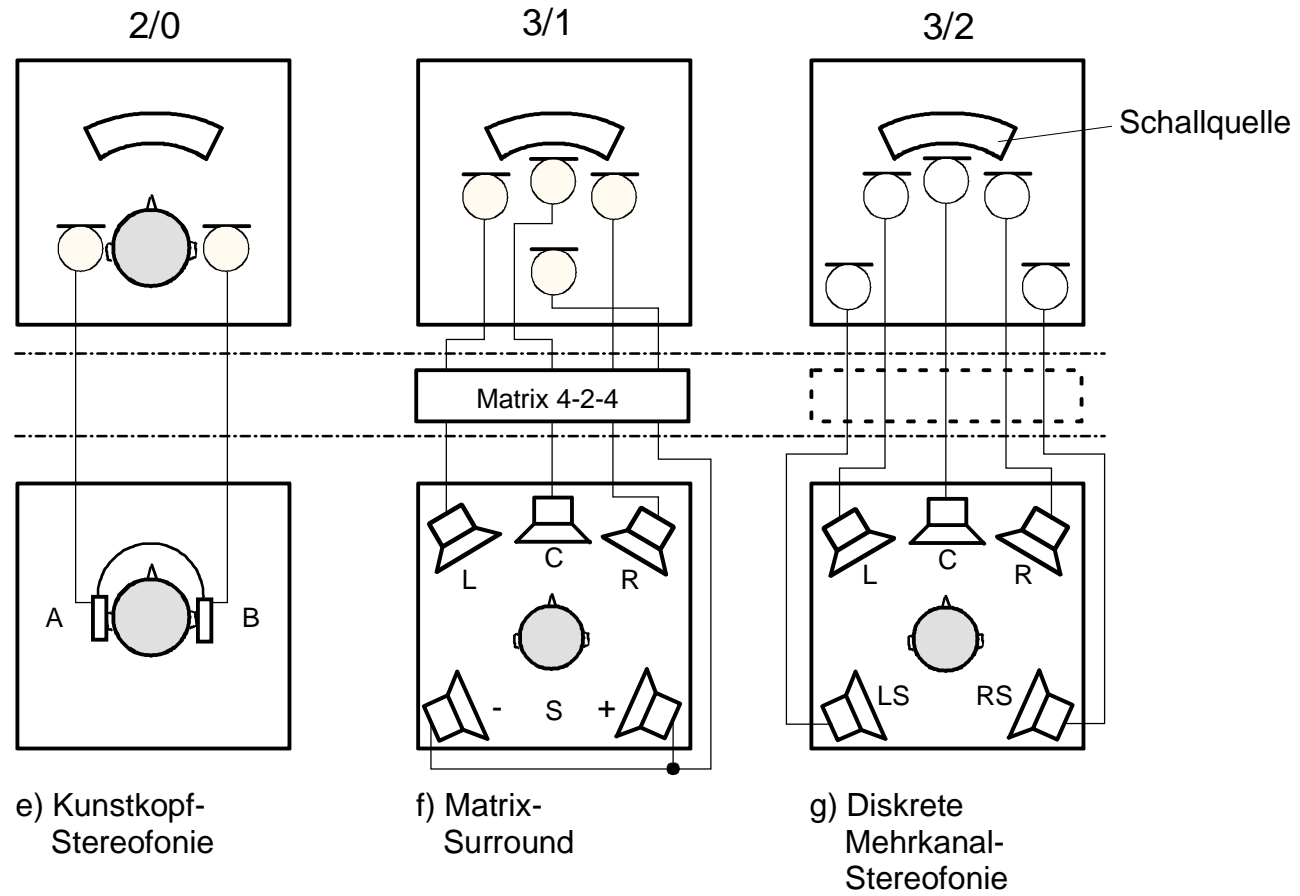
Schematische Darstellung der Übertragungsverfahren der Mehrkanalstereofonie
