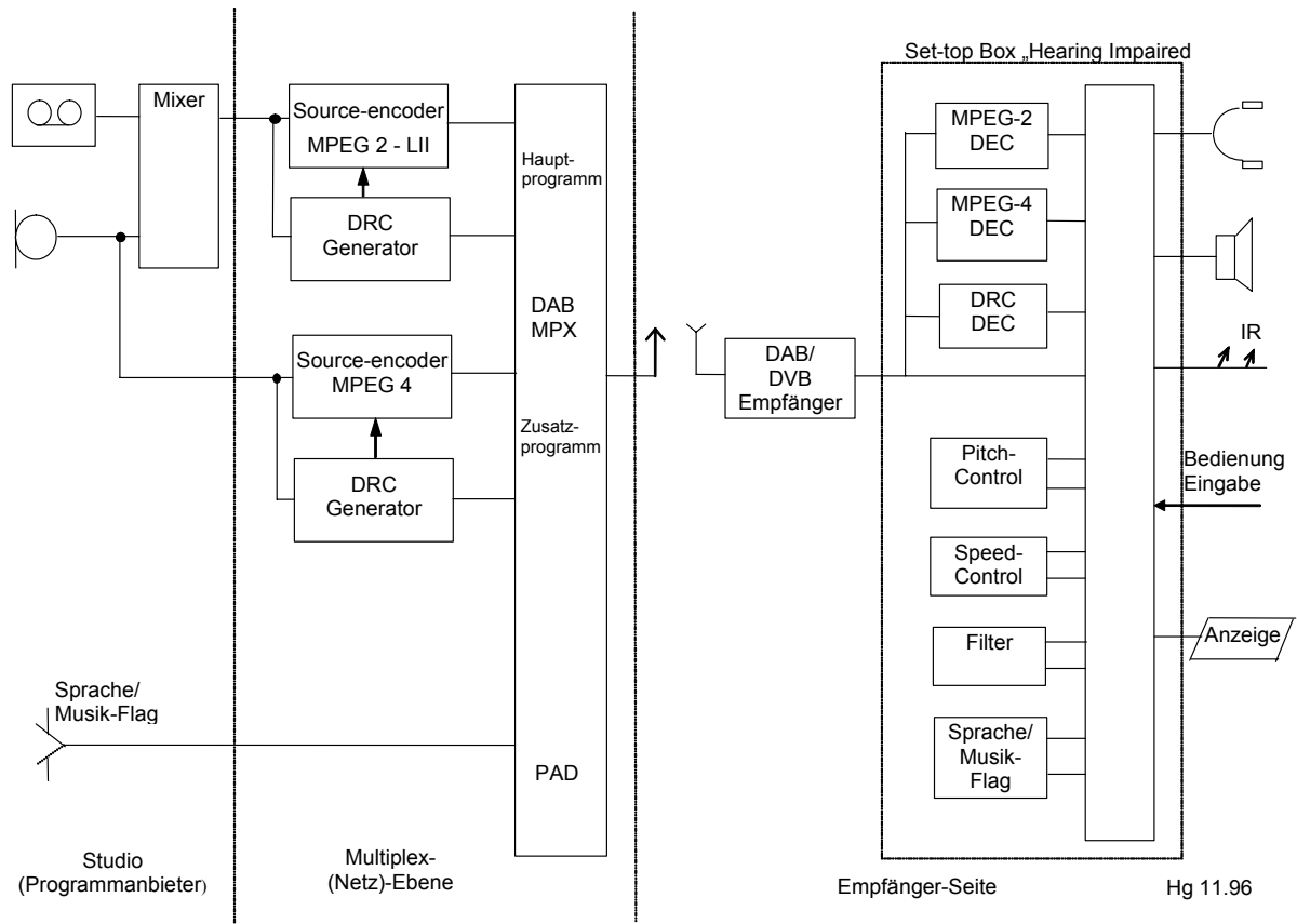
Bild 7-2 Prinzip der Tonsignalübertragung für Hörgeschädigte (Hearing impaired) bei DAB, DABplus, DMB oder DMB, nach [51]
